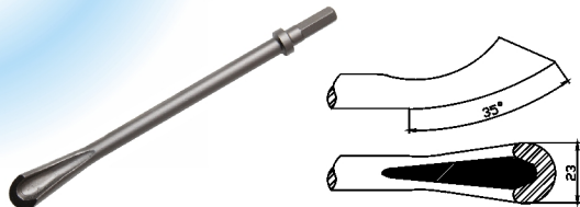
TP-2046 Hollow Gouge
