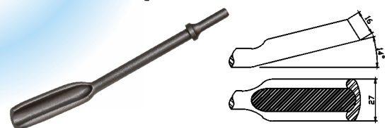
TP-2049 Hollow Gouge
